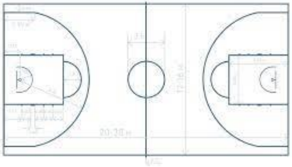
План схема розмітки баскетбольного майданчику.
